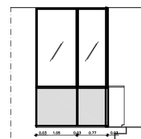
Alzato B-B Sezioni - scala 1:50
