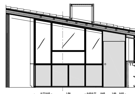
Alzato A-A
